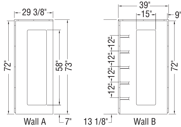
Optional Wall Set
